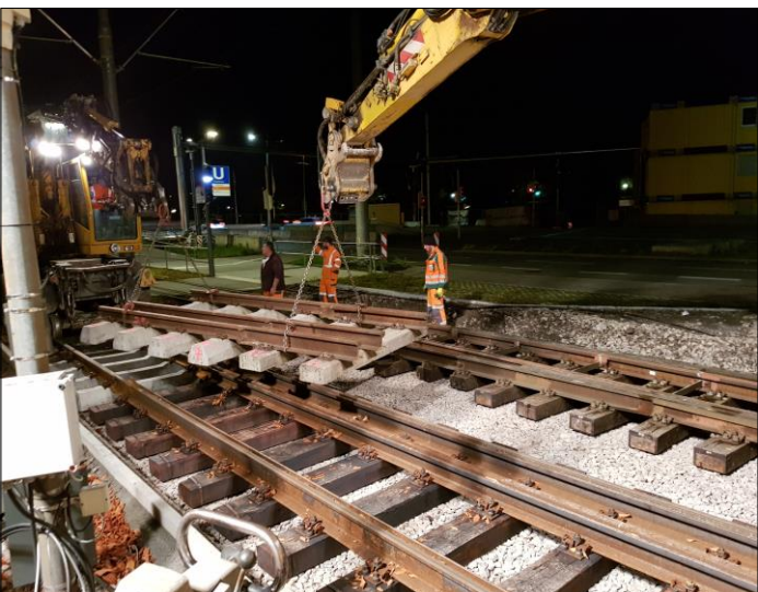
Bild 5: Einbau von Gleisrahmen
