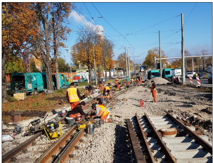
Bild 6: Verschweißen der Schienenstöße
