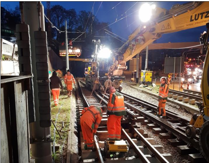
Bild 3: Einbau von Gleisrahmen
